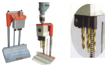
Аппарат тройного сверления
