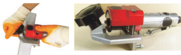
Станок для фрезерования водоотливных каналов
