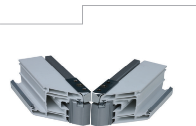
Цулага для сварочного станка
